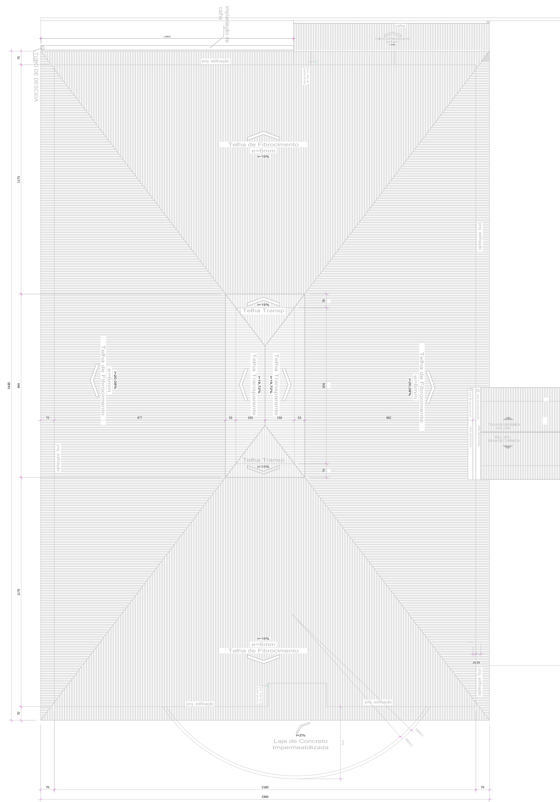
PLANTA DE COBERTURA escala 1/100
